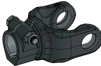
KAMALI YARIKLI KEYWAY & CLAMP BOLT MÂCHOIRE CANNELÉE AVEC BOULON TANGENT MIT KLEMMSCHRAUBE (KRAFTSCHLUSS)
